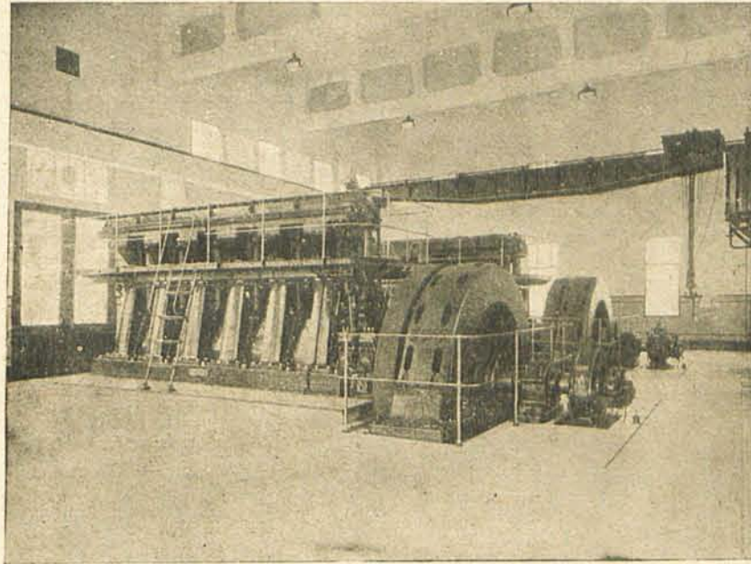
Dos grupos de 600 cab. de la Central Térmica de la Eléctrica de Orense.
