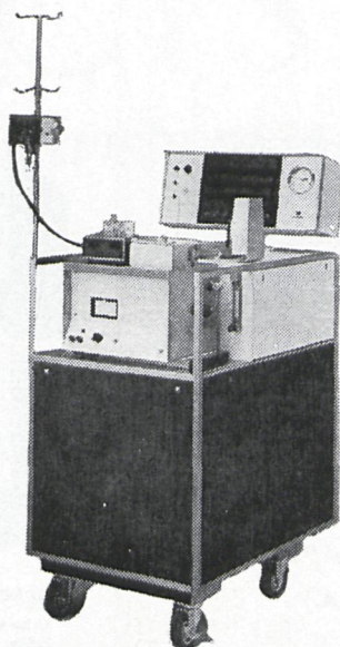
Riñón Artificial Travenol Modelo R. S. P.
