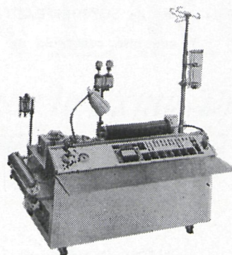
Unidad de circulación extracorpórea
