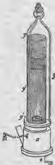
Lámpara de seguridad de Davy.
