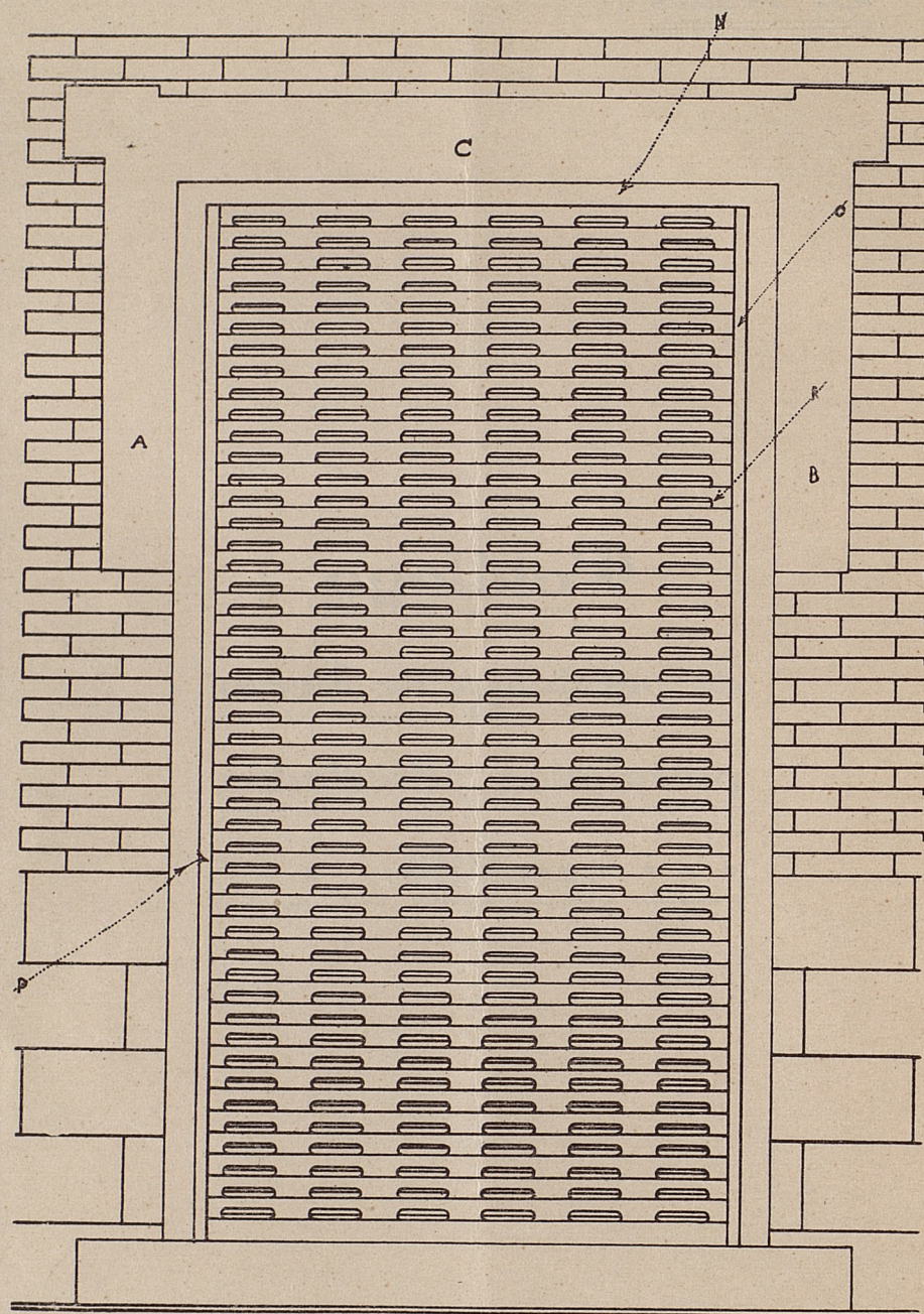
PERSIANA VISTA DE FRENTE Y CERRADA
