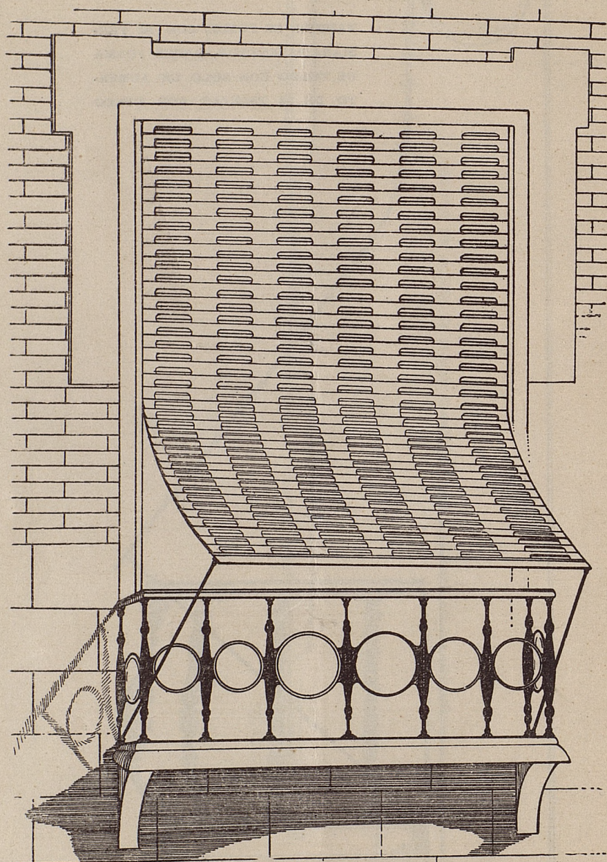
VISTA DE LA PERSIANA DE FRENTE, FORMANDO TOLDO
