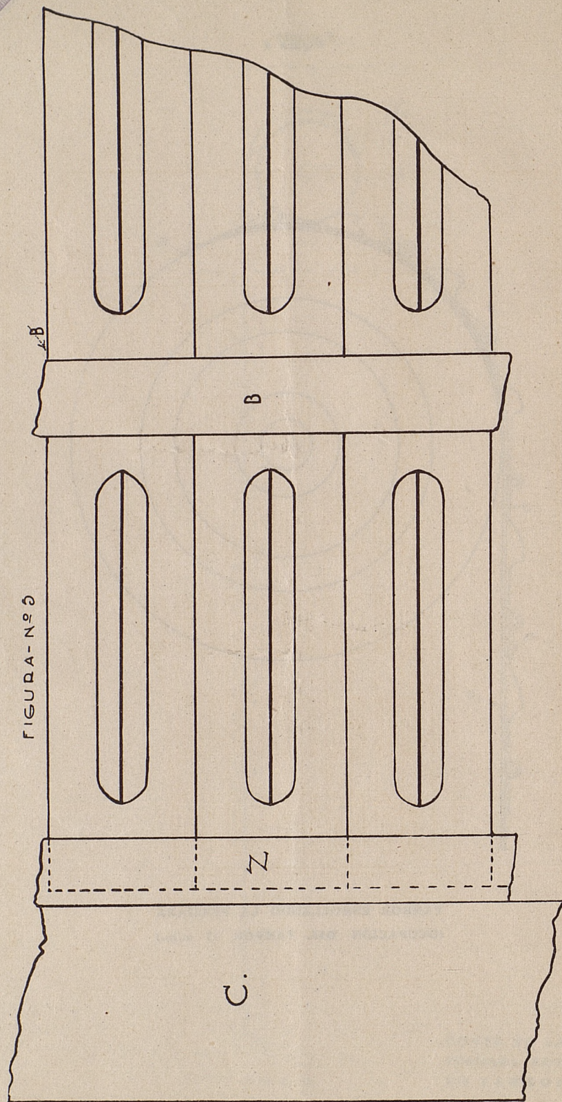
TROZO DE PERSIANA CON SU VISTA EXTERIOR
