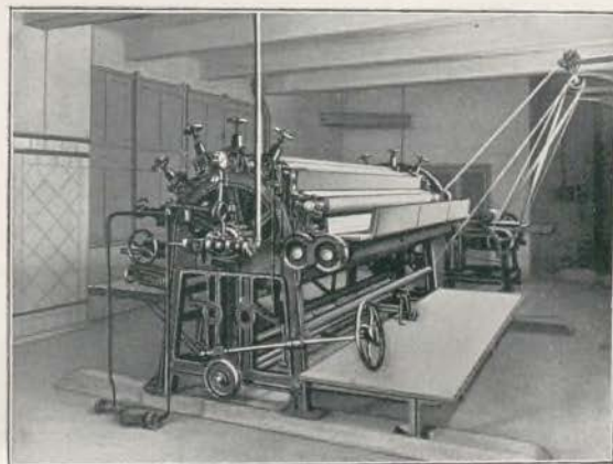
Planchadora mecánica
