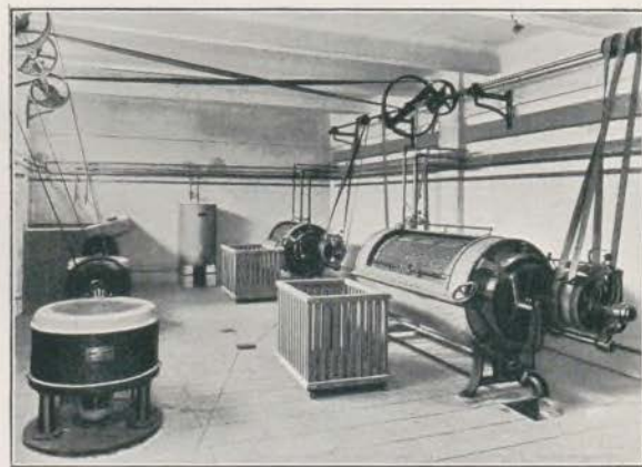
Lavadero mecánico
