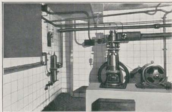
Maquinaria frigorífica
