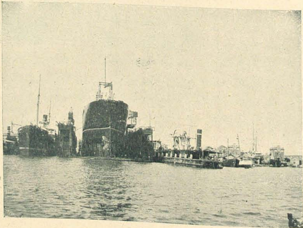
Dique flotante propiedad de "Unión Naval de Levante, S. A.", fondeado en el puerto de Valencia, con fuerza ascensional para poner en seco buques hasta de 4.200 toneladas de peso, 120 metros de eslora y manga no superior a 20 metros.
