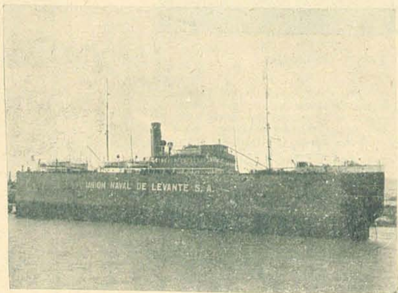
Dique flotante de 2.000 toneladas de fuerza ascensional propiedad de "Unión Naval de Levante, S. A.", fondeado en Málaga, donde cuenta con talleres para efectuar toda clase de reparaciones a flote y en seco a buques de guerra y mercantes.
