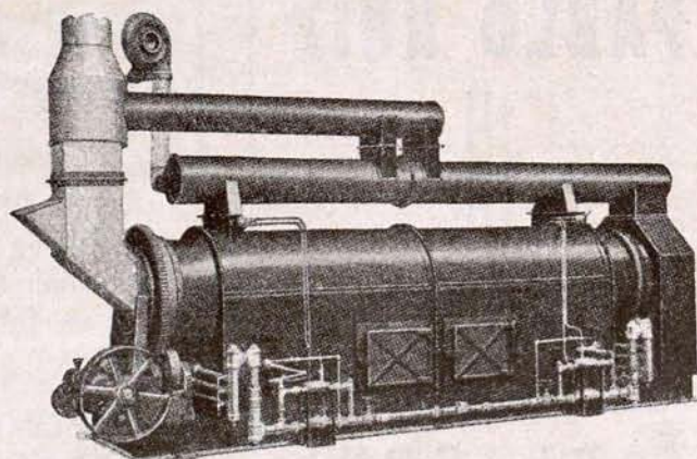
Secador rotatorio calentado por gas.
