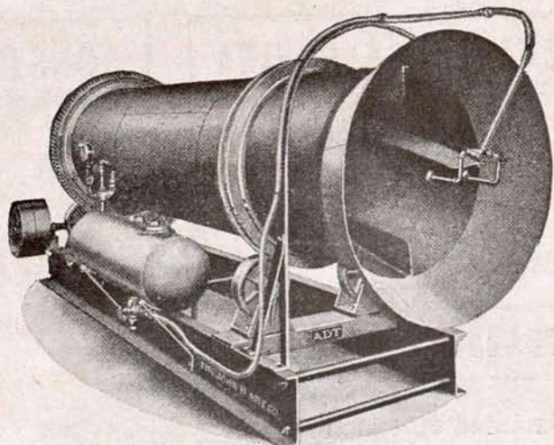
Cilindro aromatizador.
