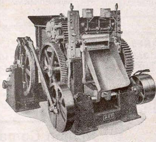
Máquina de cortar tabaco.
