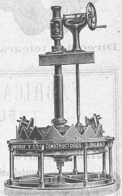
TURBINA EN POZO ABIERTO PARA PEQUEÑOS SALTOS
