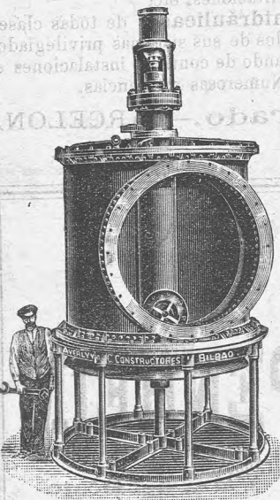
TURBINA DE 200 CABALLOS CONSTRUIDA PARA LA SOCIEDAD ANÓNIMA ALAMBRES DEL CADAGUA BILBAO FUNDICION
