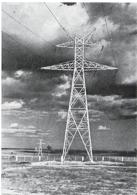
Torre de conducción a 132 KV.
