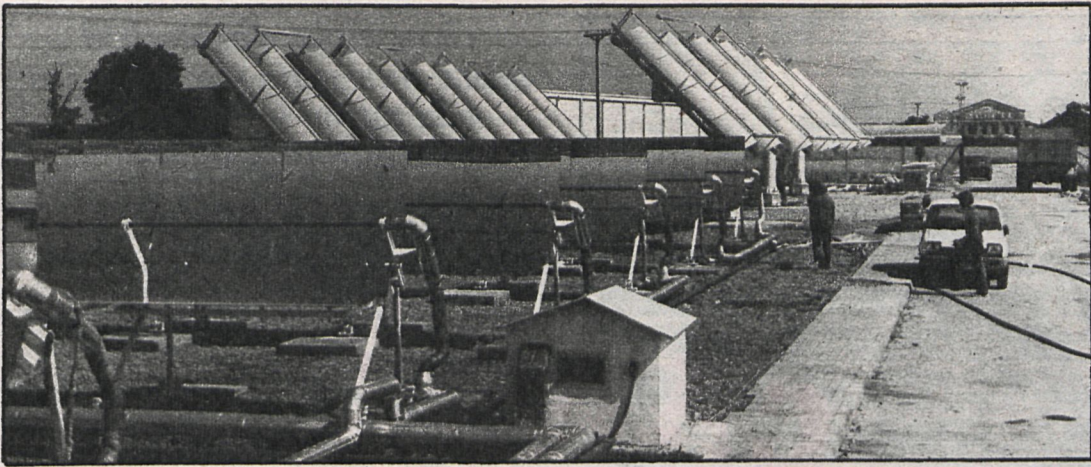
La granja solar de Getafe tiene una potencia de 250 KW térmicos
