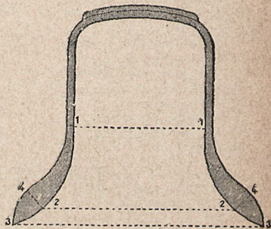
Figura 2. a —Diagrama indicador de las partes que se deben atacar para subir ó bajar el tono de una campana.
