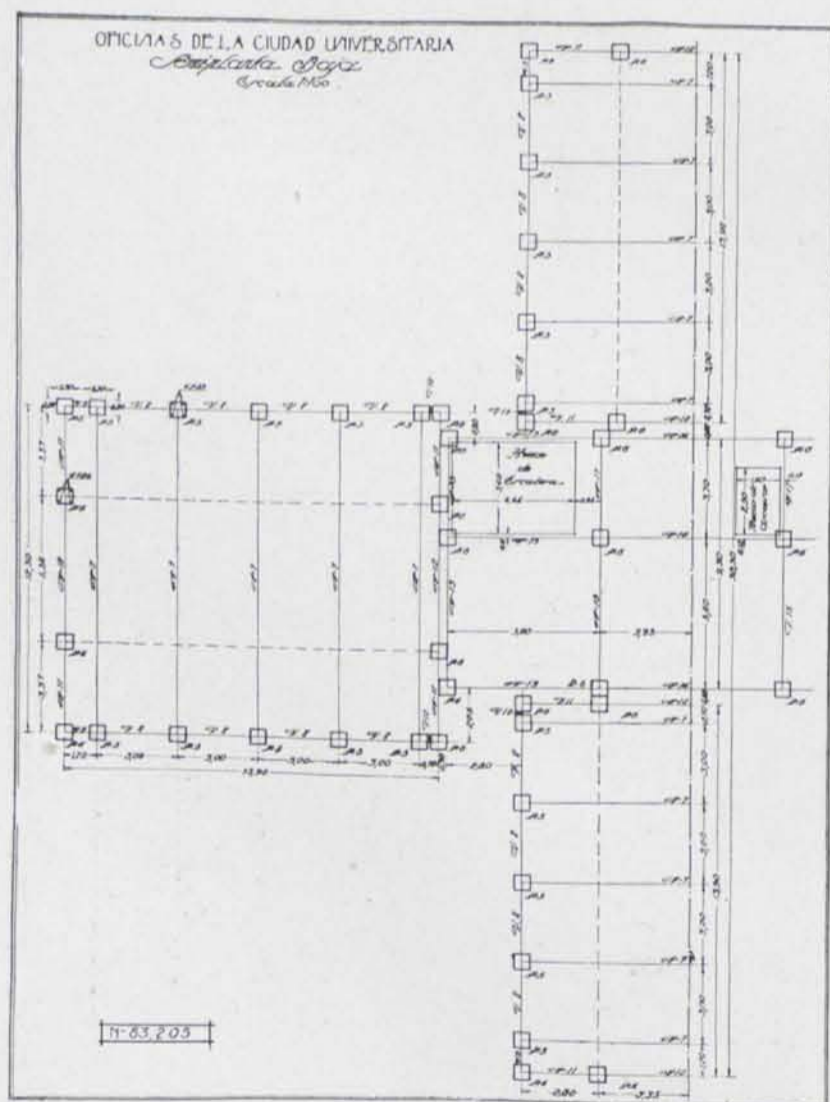
Planta de pilares.
