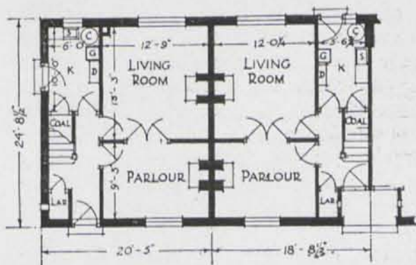
Planta baja.
