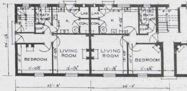
Planta baja.
