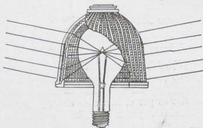
1. Aparato refractor para alumbrado público.
