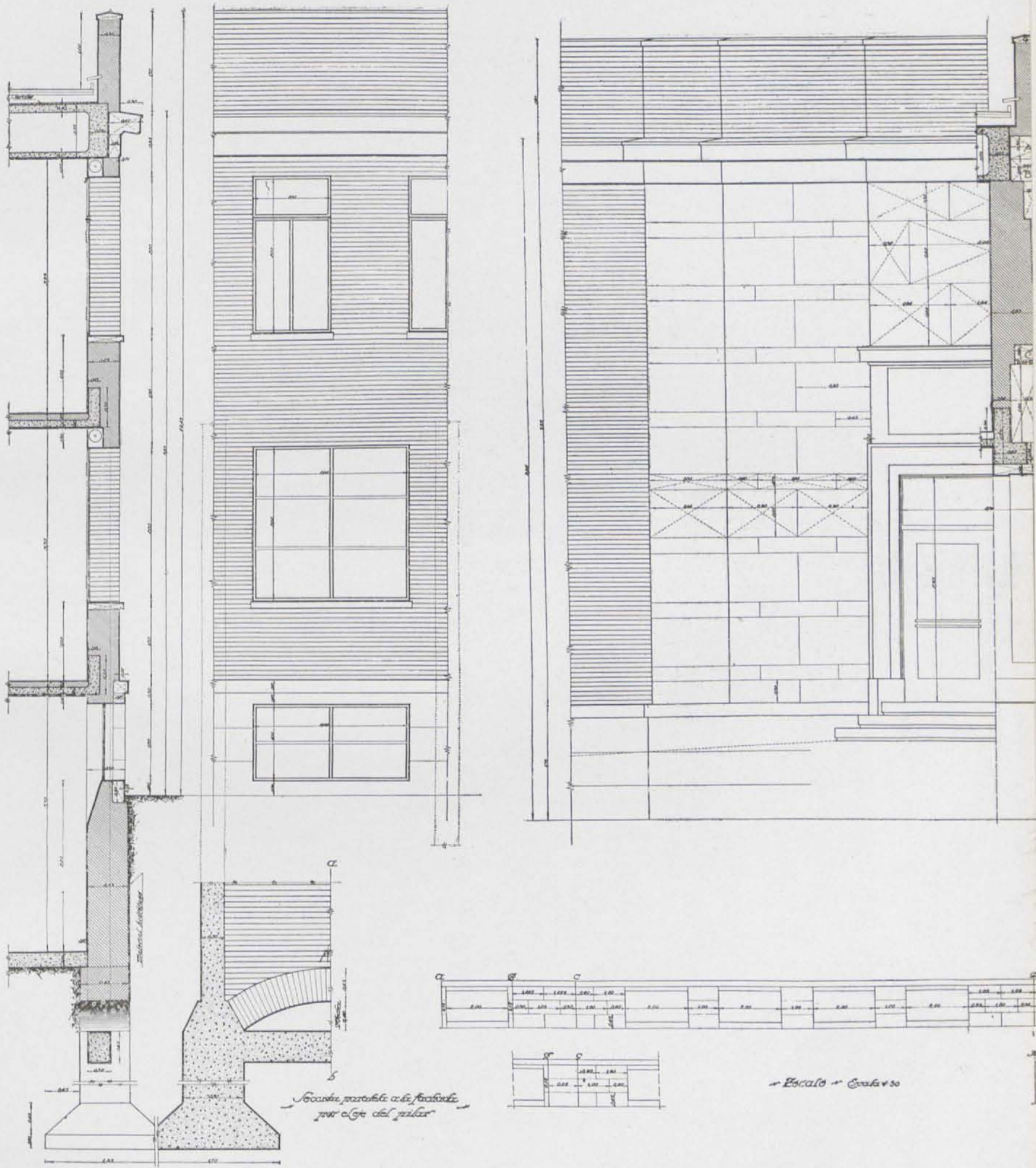
Pabellón y Oficinas de la Ciudad Universitaria. (Detalles.)
