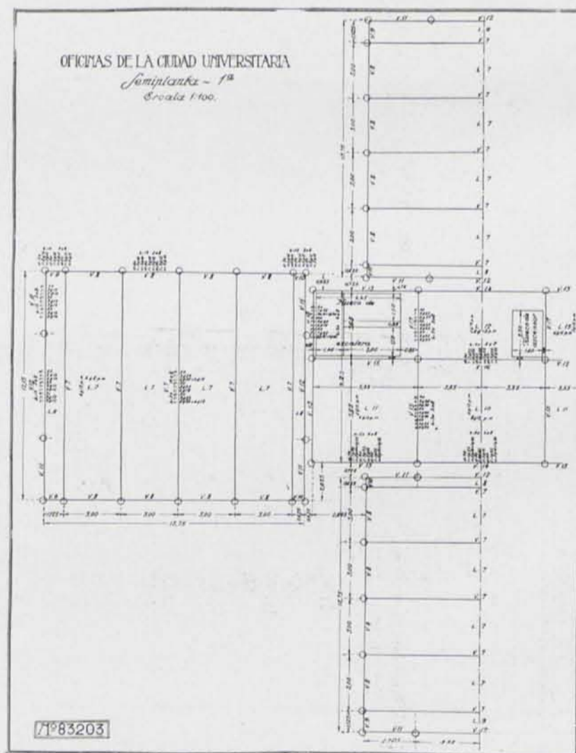
Planta de vigas y tableros.
