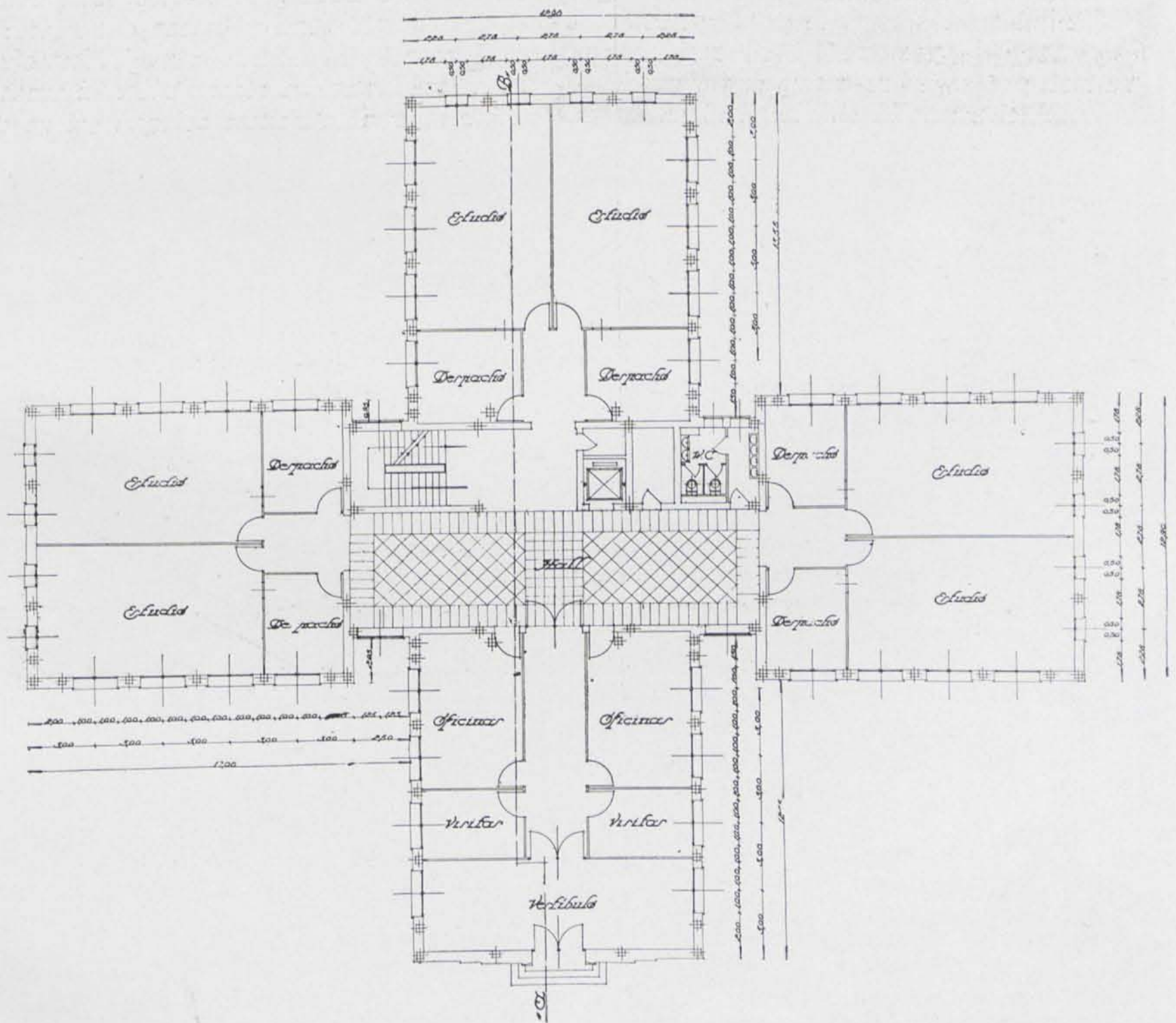
Planta baja.
