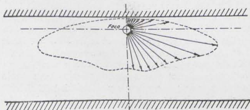
2. Curva asimétrica de distribución de luz.
