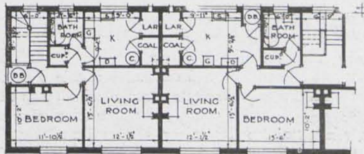
Planta alta.
