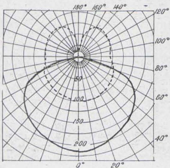
6. Curva fotométrica de aparato simétrico.
