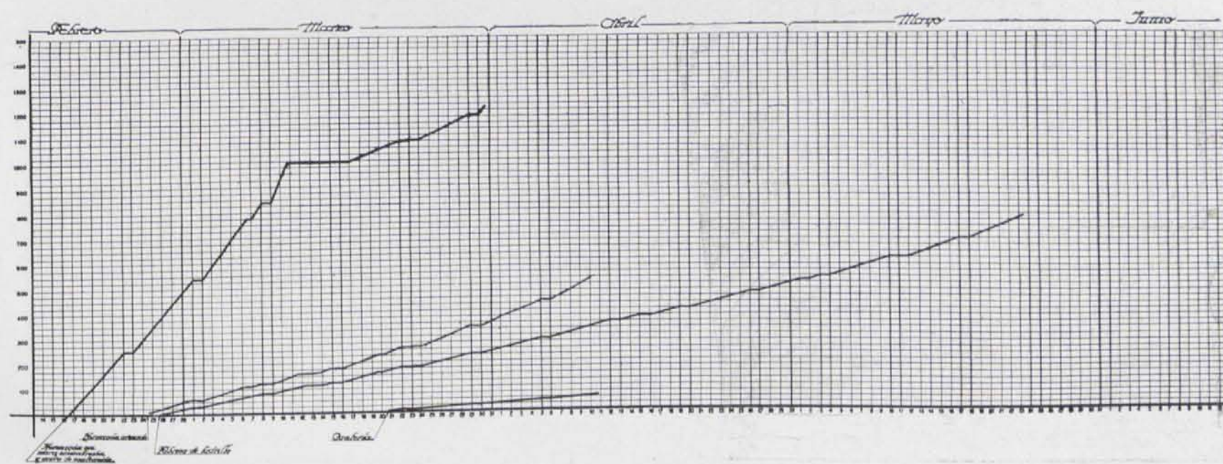
Gráfico de marcha de los trabajos.
