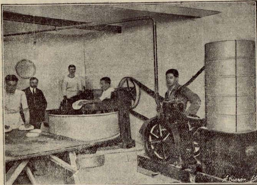
El obrador donde se hace el PAN BOMBÓN: Motor y parte de la maquinaria
