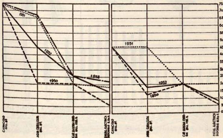
GRÁFICO DE CAPACIDAD DE ENERGIA Y AGUA EMBALSADA
