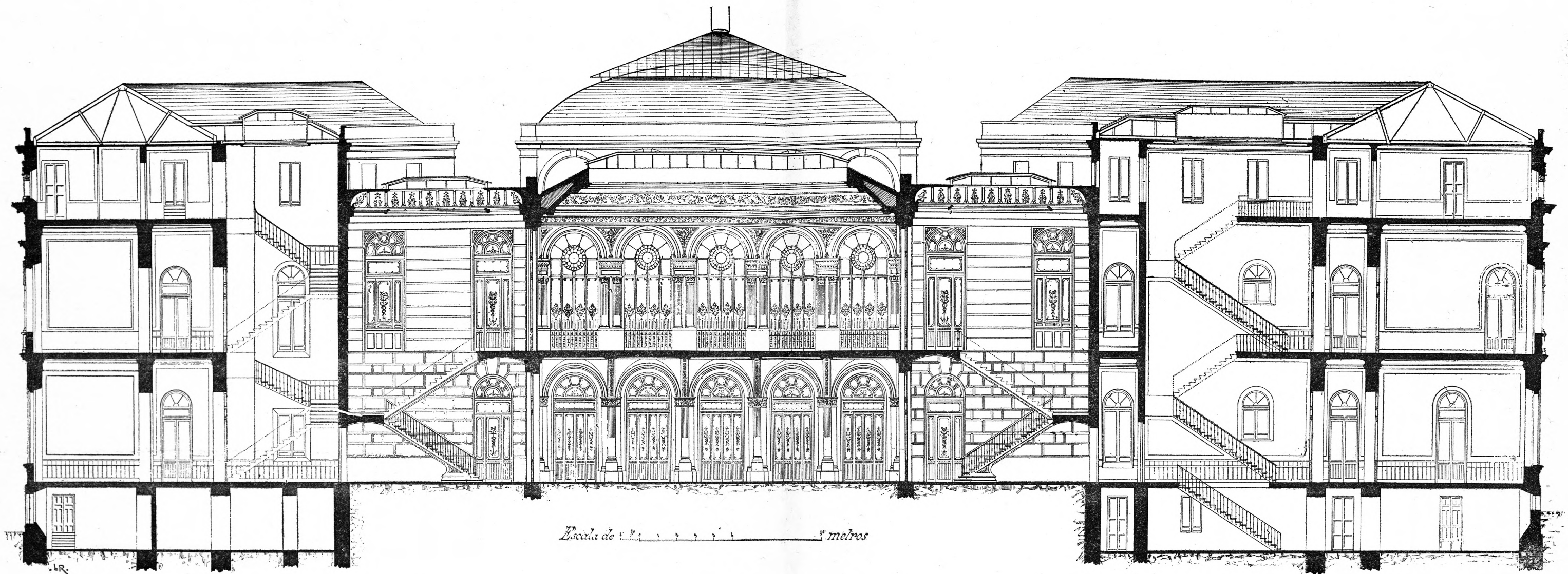
SECCIÓN TRANSVERSAL
