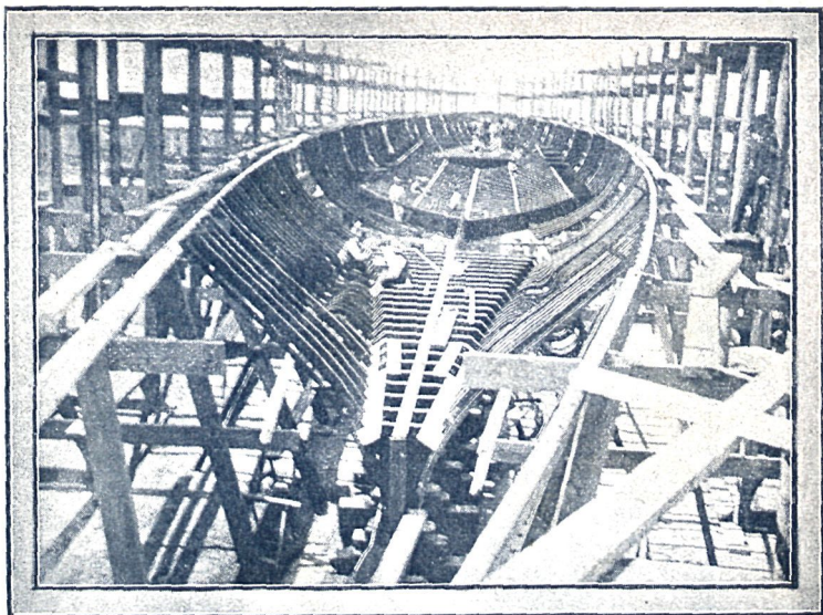
CÁDIZ: CRUCERO «EXTREMADURA» EN CONSTRUCCIÓN EN LOS ASTILLEROS DE LA «CONSTRUCTORA NAVAL ESPAÑOLA»
