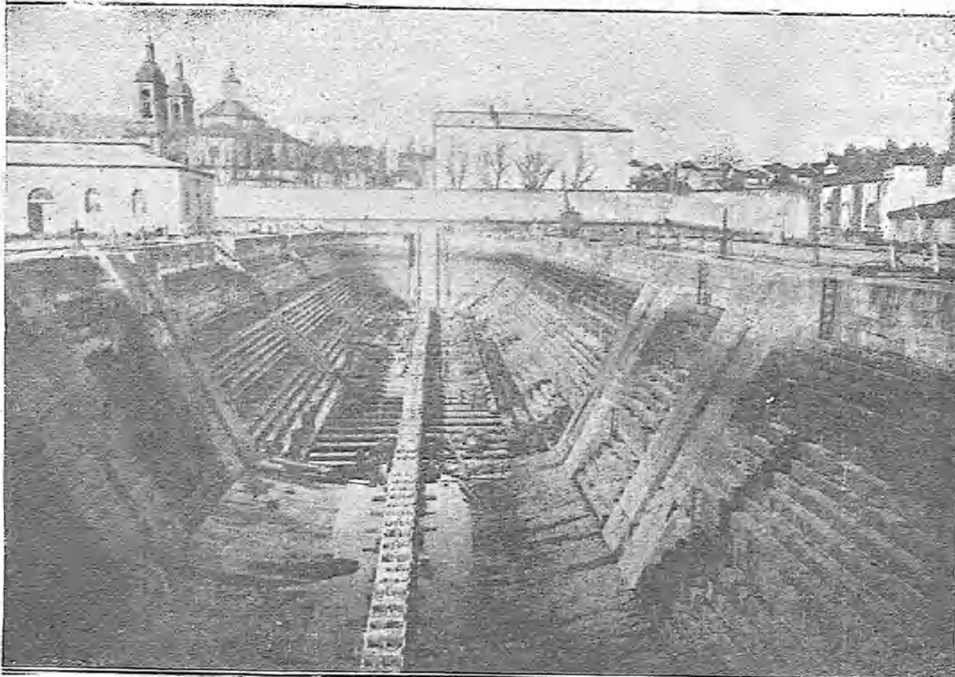
DIQUE DE LA CAMPANA EN EL ARSENAL DEL FERROL (Fots. S. Linares.)
