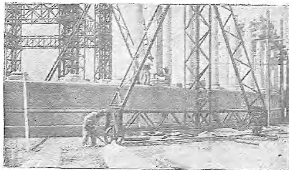
LA GRÚA GIGANTESCA DEL SR. GRASES, DESTINADA Á ELEVAR LAS COLUMNAS
