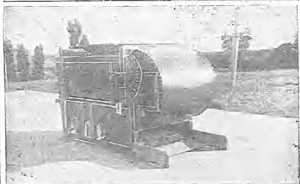
AVENTADORA MOVIDA A BRAZO. PRESENTADA POR DON FRANCISCO JIMÉNEZ Y COMPAÑÍA, DE VALLADOLID, QUE OBTUVO EL SEGUNDO PREMIO (C.ols. de Góñ.)
