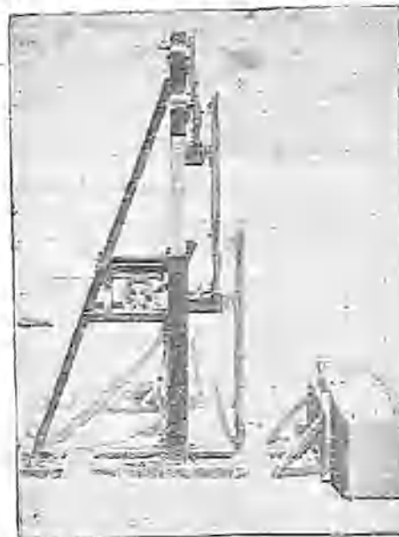
PERIL DEL CABALLETE QUE SOSTIENE LAS PLANCHAS
