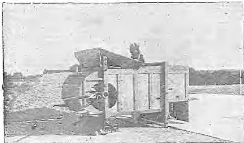
AVENTADORA MOVIDA POR MALACATE. PRESENTADA POR LA CASA DE DON ANTONIO CUITAT, DE LERIDA, QUE OBTUVO LA PRIMERA RECOMPENSA
