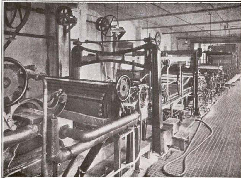
Vista general de una de las máquinas planas que fabrican el papel de fumar «Smoking».
