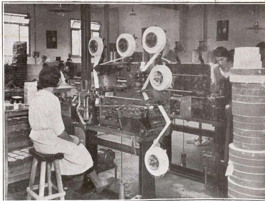
Máquinas que fabrican los blocks «Smoking» de 500 hojas timbradas y engomadas, al tamaño de la máquina Victoria.
