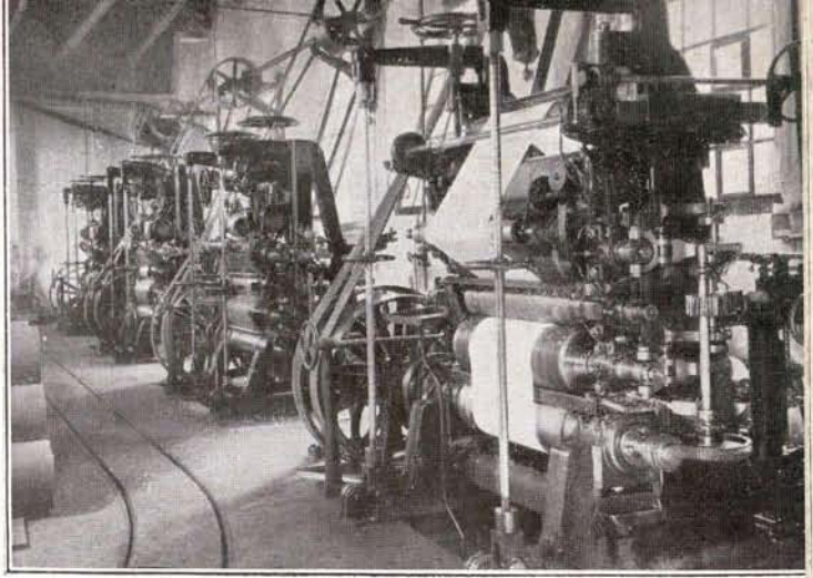
Sala de máquinas filigranadoras, en donde se marca el papel a presión.
