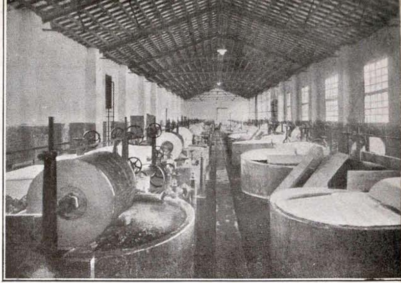
Vista de una isla de cilindros en los que se prepara la pasta.
