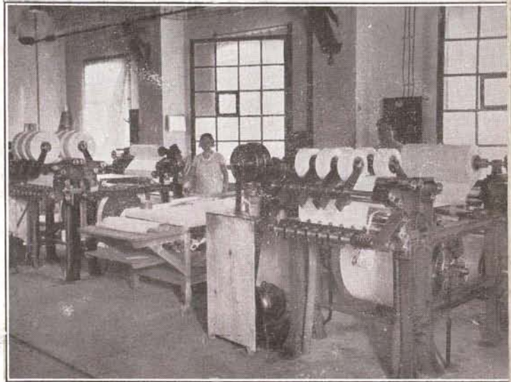
Máquinas que engoman con goma vegetal el borde del papel destinado a la fabricación del estuche «Smoking».
