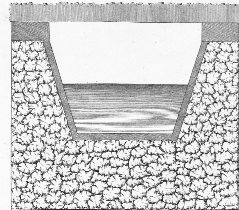
Perfil del Acueducto reunido
