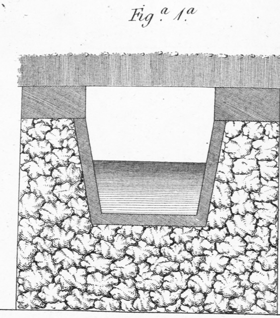
Perfil del Acueducto de Guadalupe
